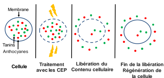
Figure N°1 : Principe de l'électroporation
