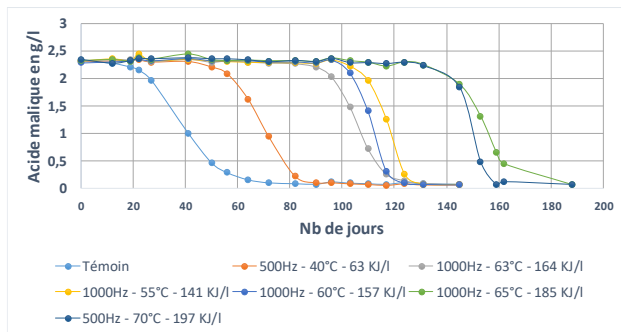
Figure N°13 : Tests de stabilisation microbienne des vins vis-à-vis des bactéries lactiques – Recolonisation en bactéries lactiques par le suivi de la dégradation de l'acide malique
