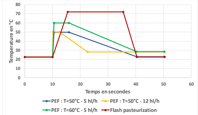
Figure N°8 : Comparaison du profil de température durant le traitement du vin par des CEP à 5 et 12 hl/l et la flash pasteurisation
