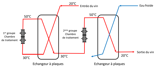
Figure N°7 : Démonstrateur de stabilisation microbienne des vins par des CEP (chambres de traitement + générateur) couplé à un échangeur de chaleur à plaques
