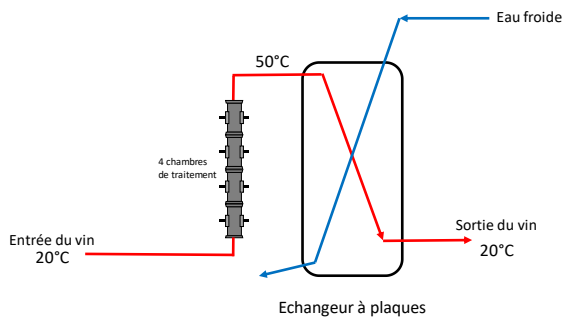
Figure N°5 : Montage des 4 chambres de traitement en série avec refroidissement par un échangeur à plaque
